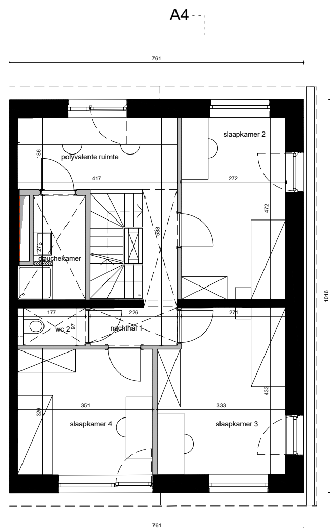
NIVEAU +1
