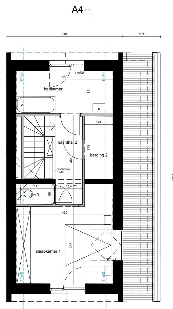
NIVEAU +2
