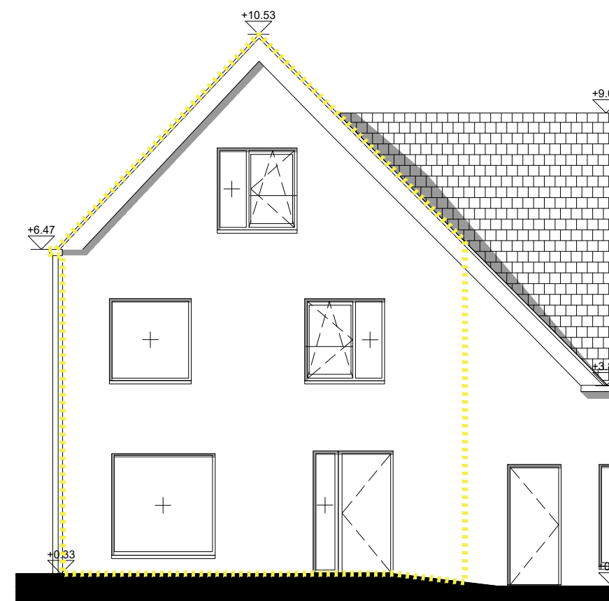
NOORD GEVEL
