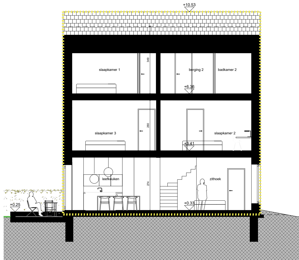
SNEDE A4
