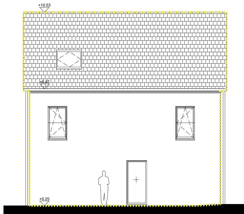
OOST GEVEL
